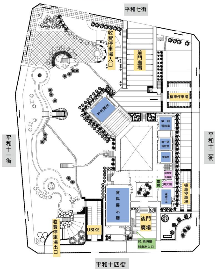
一樓平面圖
