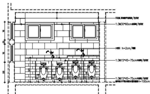
2 E剖面圖 A3:S=1/40
