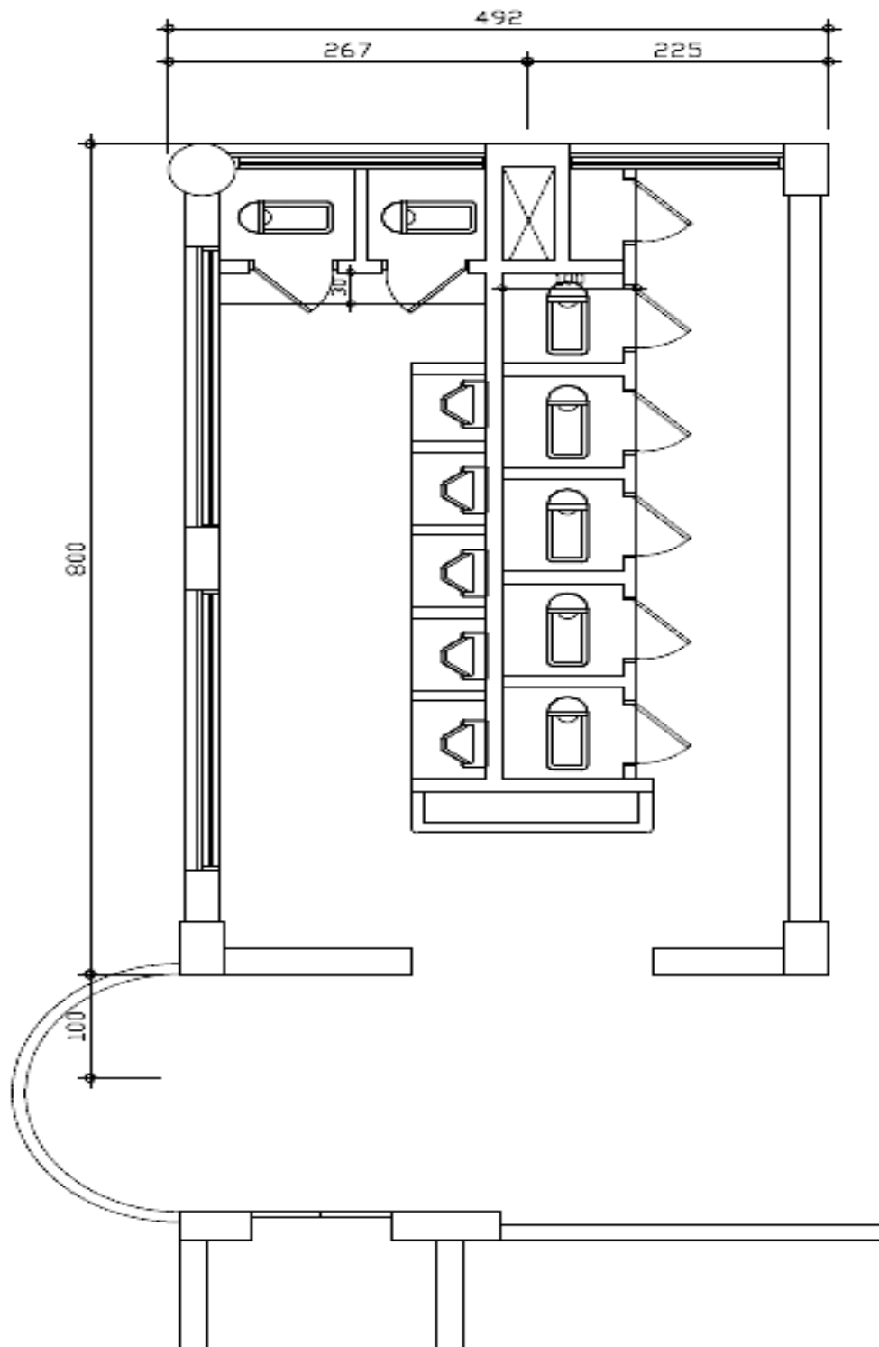
南棟西側三樓平面圖
