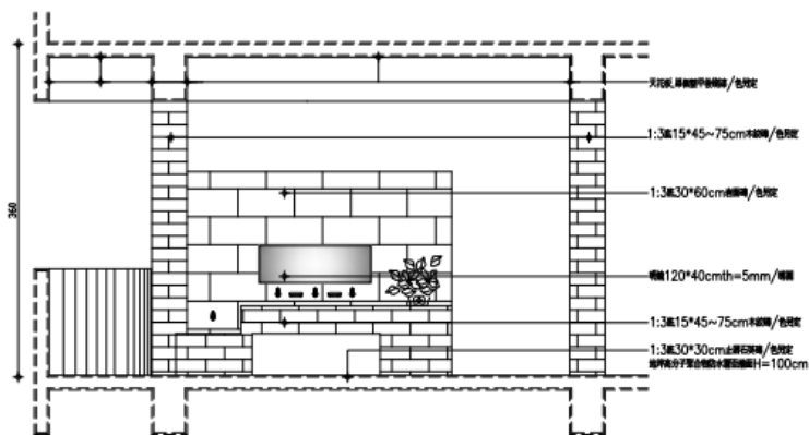
1 A剖面圖 A3:S=1/40
