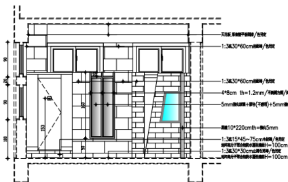
2 D剖面圖 A3:S=1/40
