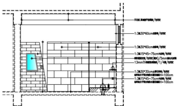
3 C剖面圖 A3:S=1/40
