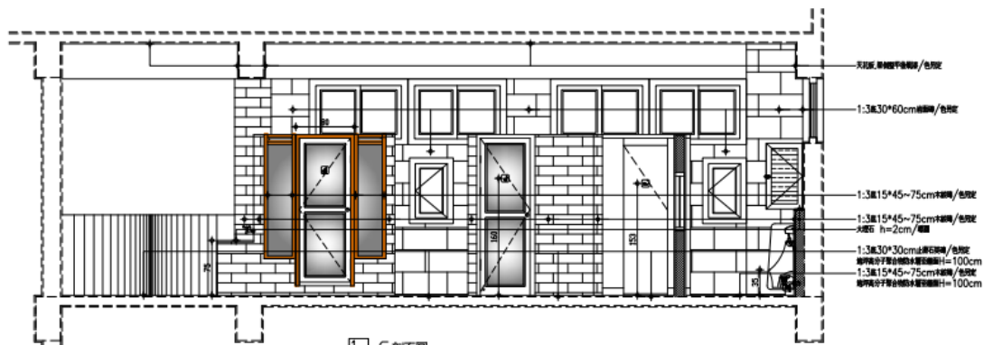
1 G剖面圖 A3:S=1/40
