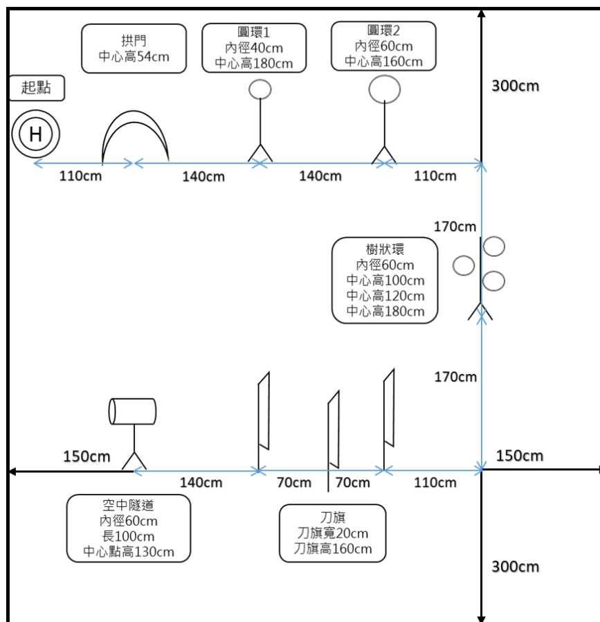
圖 1-1 競賽場地平面示意圖
