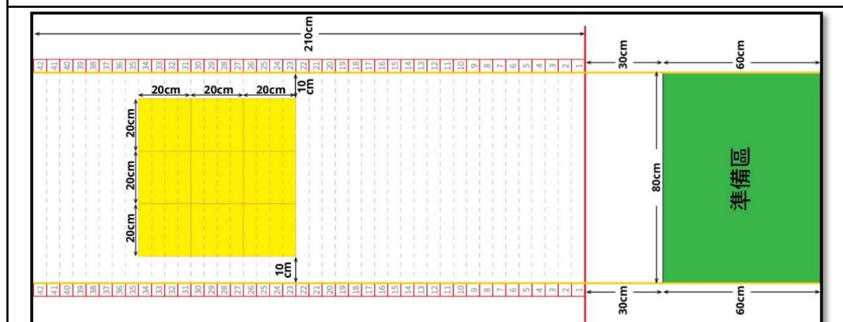
圖 9-3 競賽用場地尺寸標示
